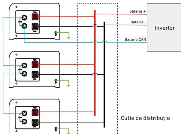
Figura 4-1 Conectarea în paralel a trei acumulatoare
