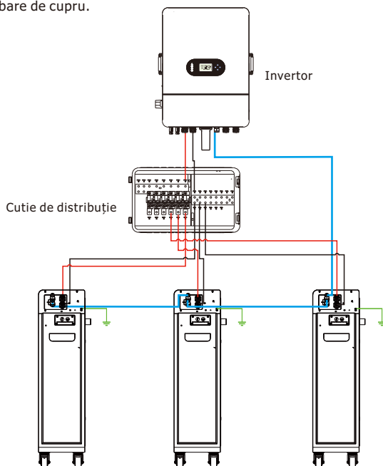
Figura 4-1 Conectarea în paralel a trei acumulatoare
